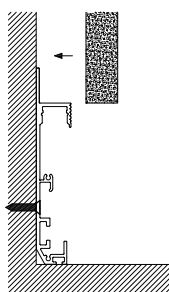
Step 02 Fix the drywall
